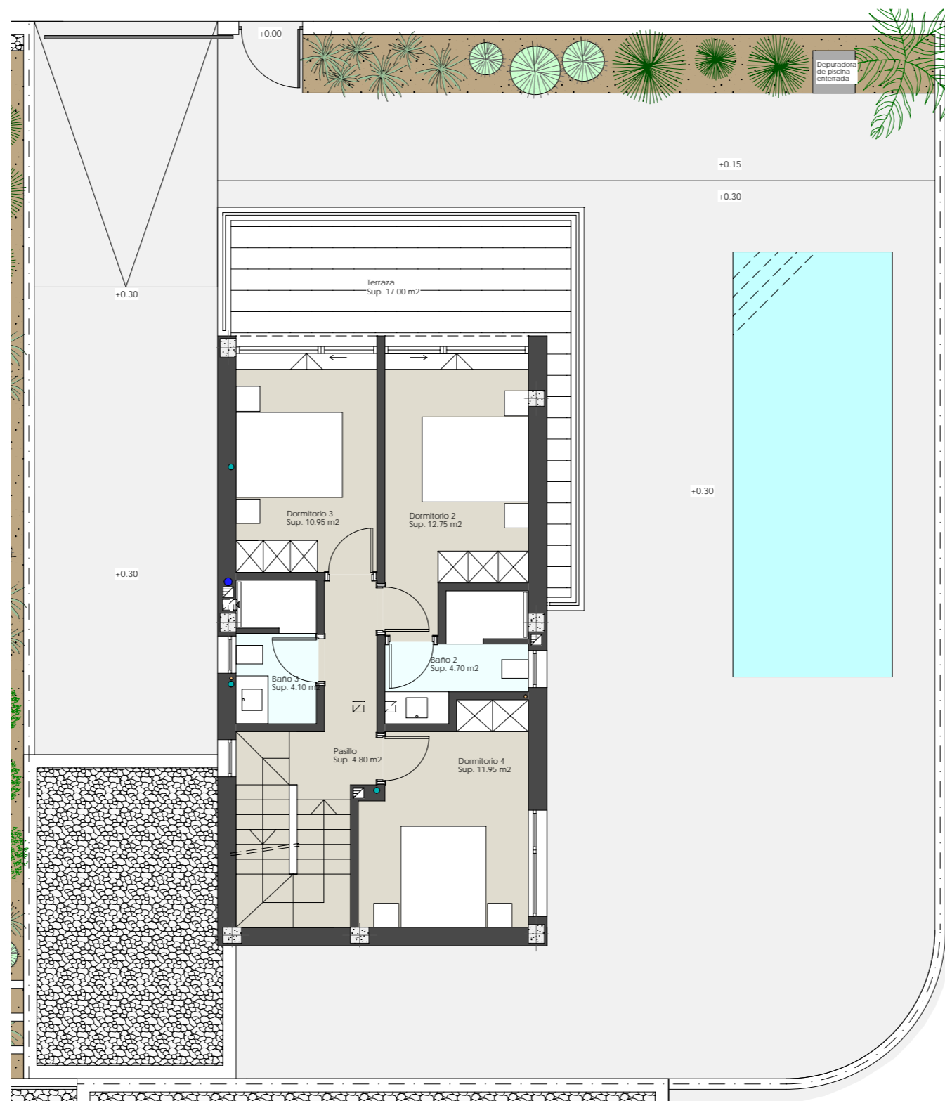
Planta primera
