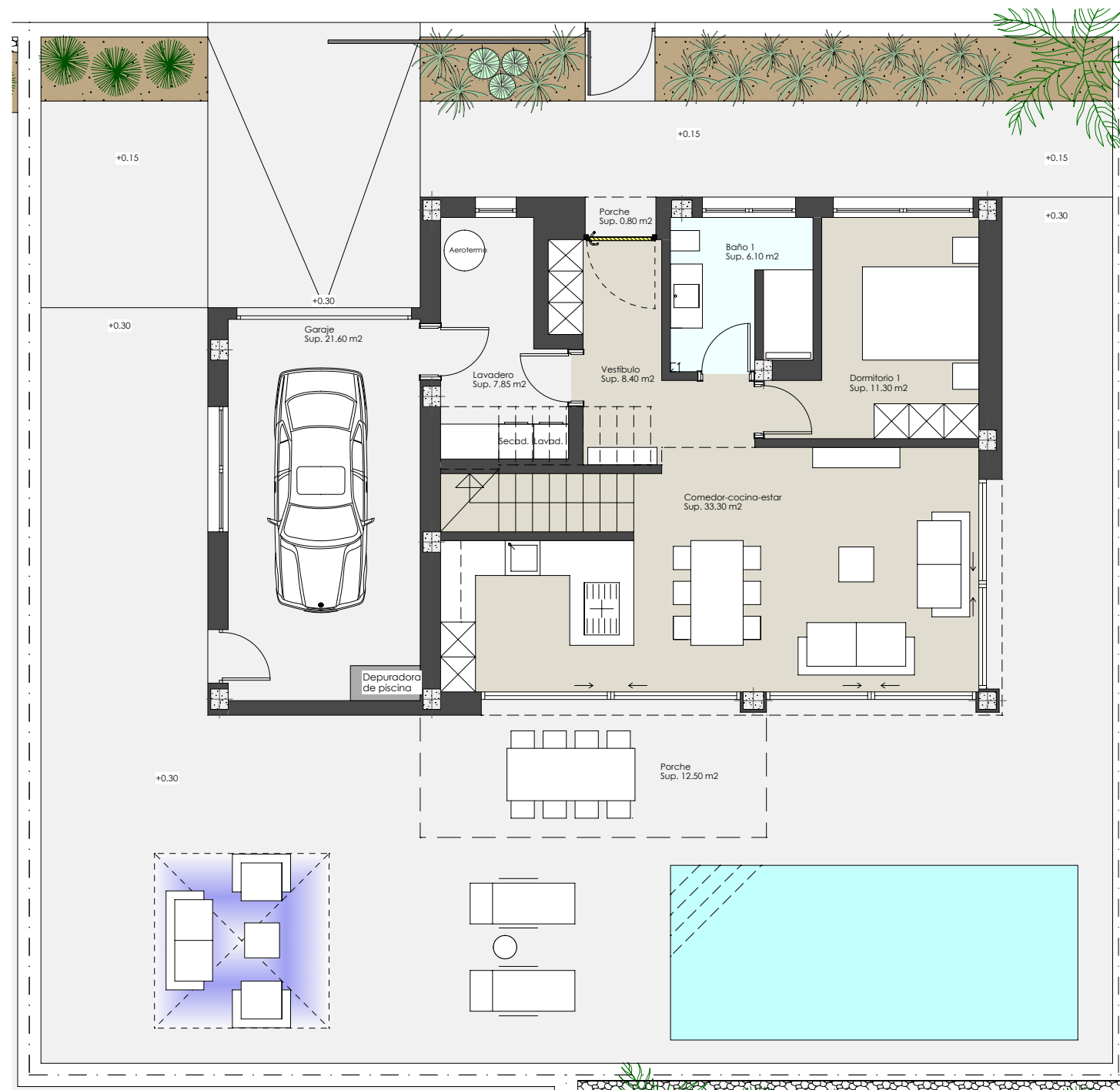
Planta baja
